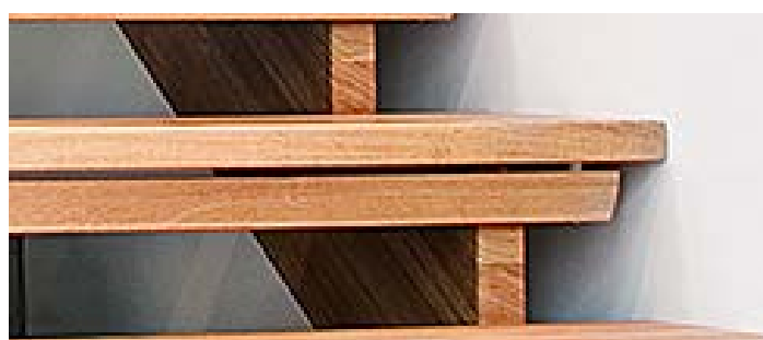
I en öppen trappa monteras en list under varje plansteg för att förhindra att barn kan tränga sig igenom och fastna.
