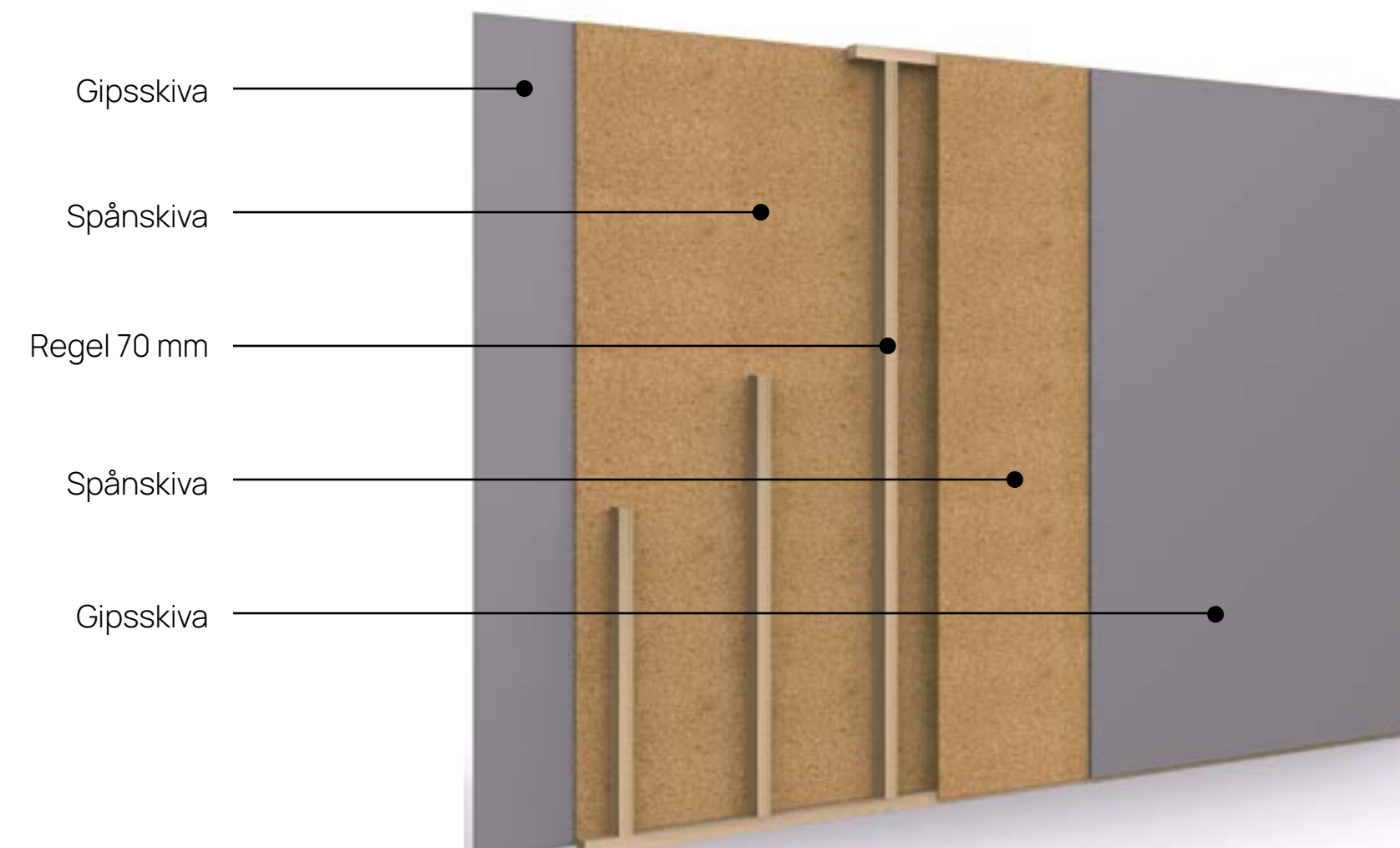
Dubbla skivor ingår i alla innerväggar
