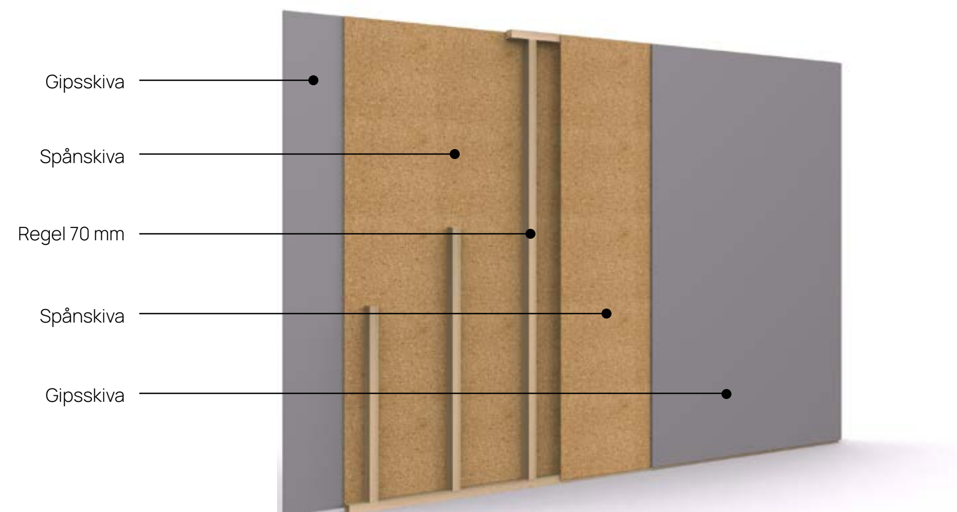
Dubbla skivor ingår i alla innerväggar
