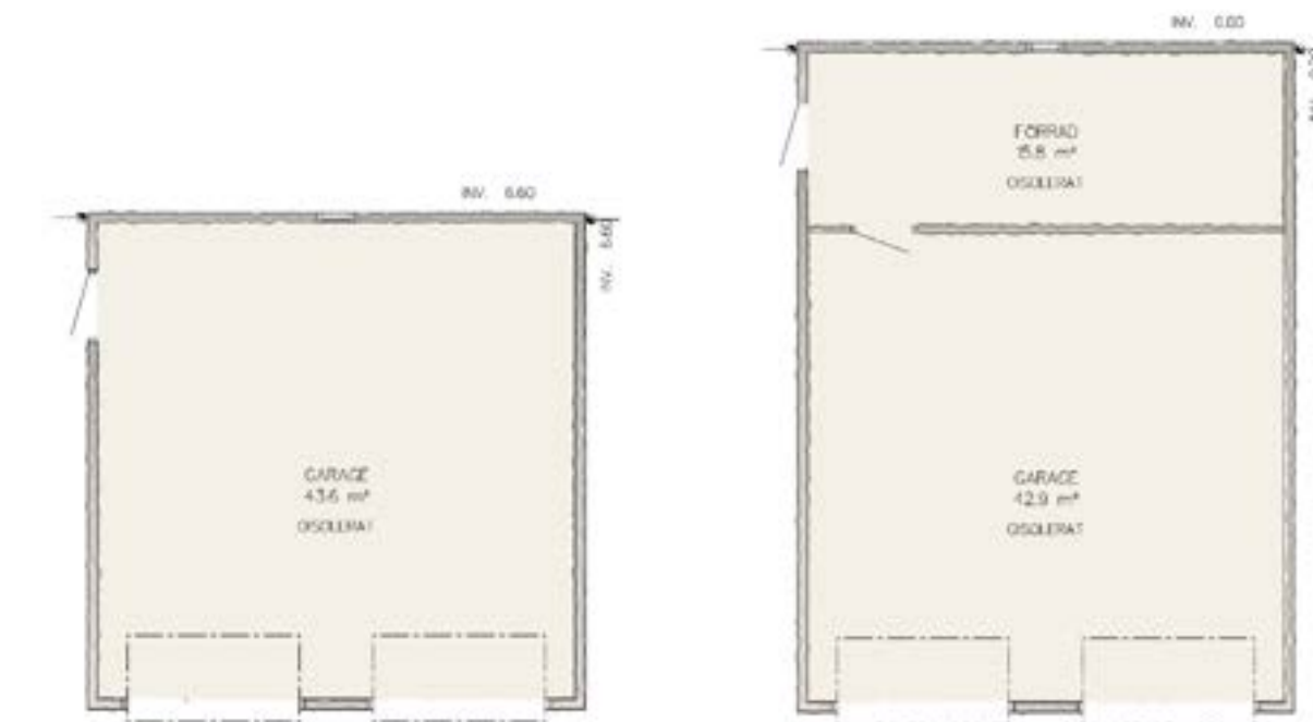
Dubbelgarage 43,6 kvm Dubbelgarage 43,6 kvm plus förråd 15,8 kvm
