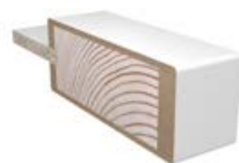
Snitt på massiv innerdörr Unique
